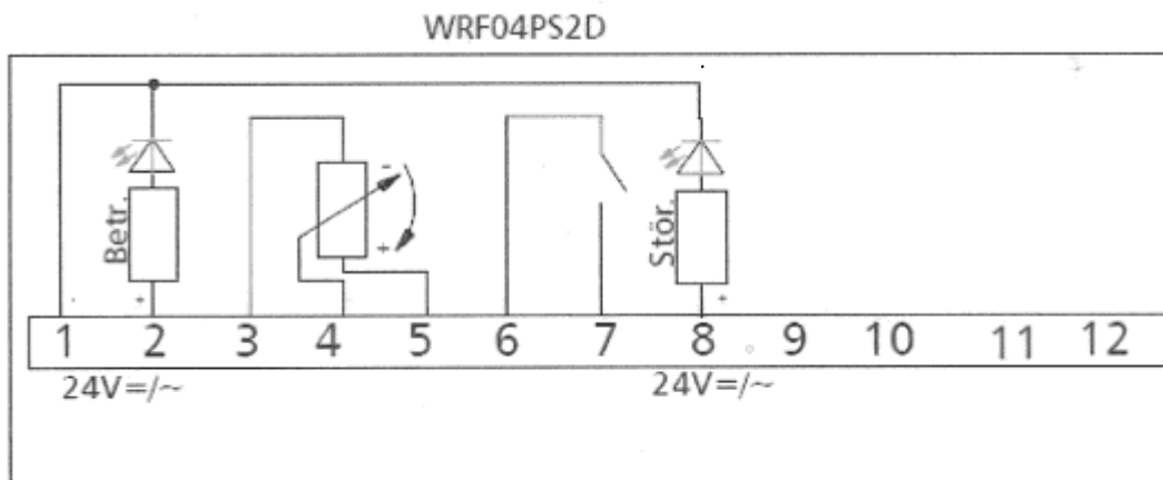
Afb. 9 Wandbediening aansluitschema, aangegeven in de wandbediening.
