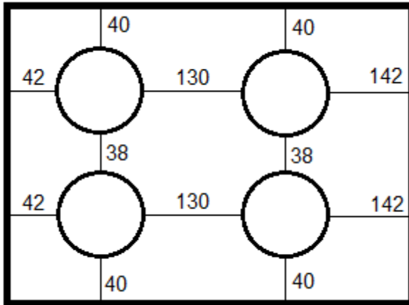
Afb. 8 bovenaanzicht Coanda®.
